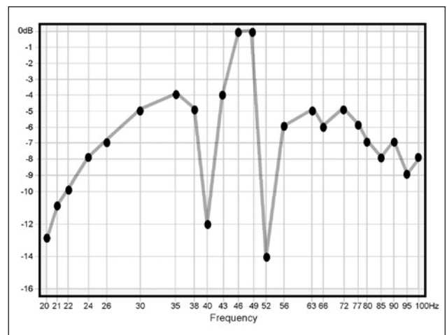
Afbeelding 19. Voorbeeld met twee nauwe dips
