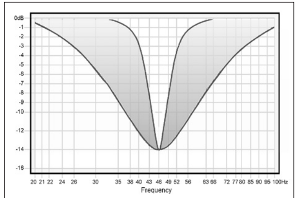
Afbeelding 11. Effect instelbare bandbreedte
