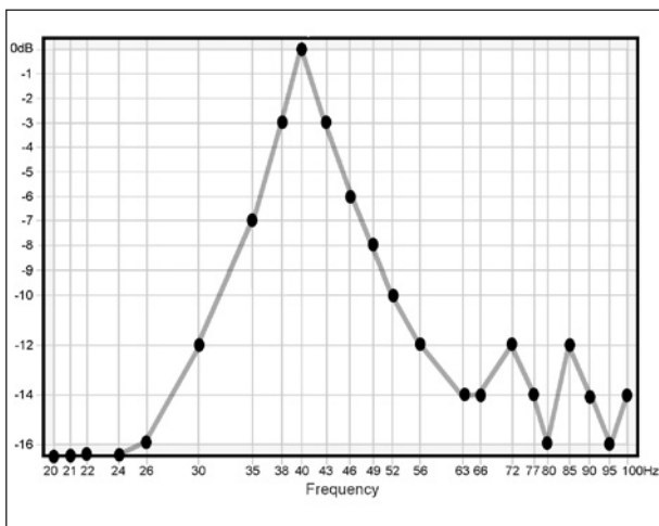
Afbeelding 18. Nauwe piek
