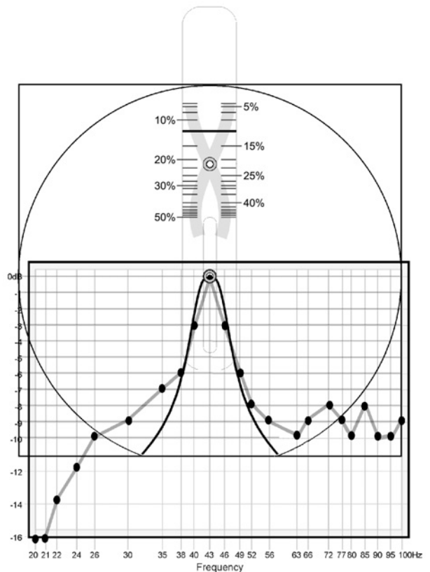
Afbeelding 14. Selector ingesteld op 'optimaal samenvallen'
